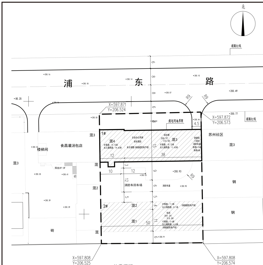
总平面图 1:500
